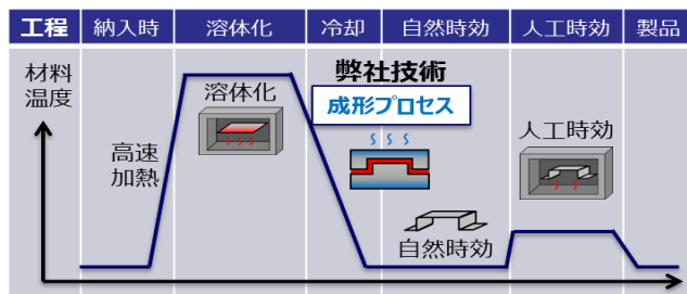
<自動車のドアインナーパネル>
